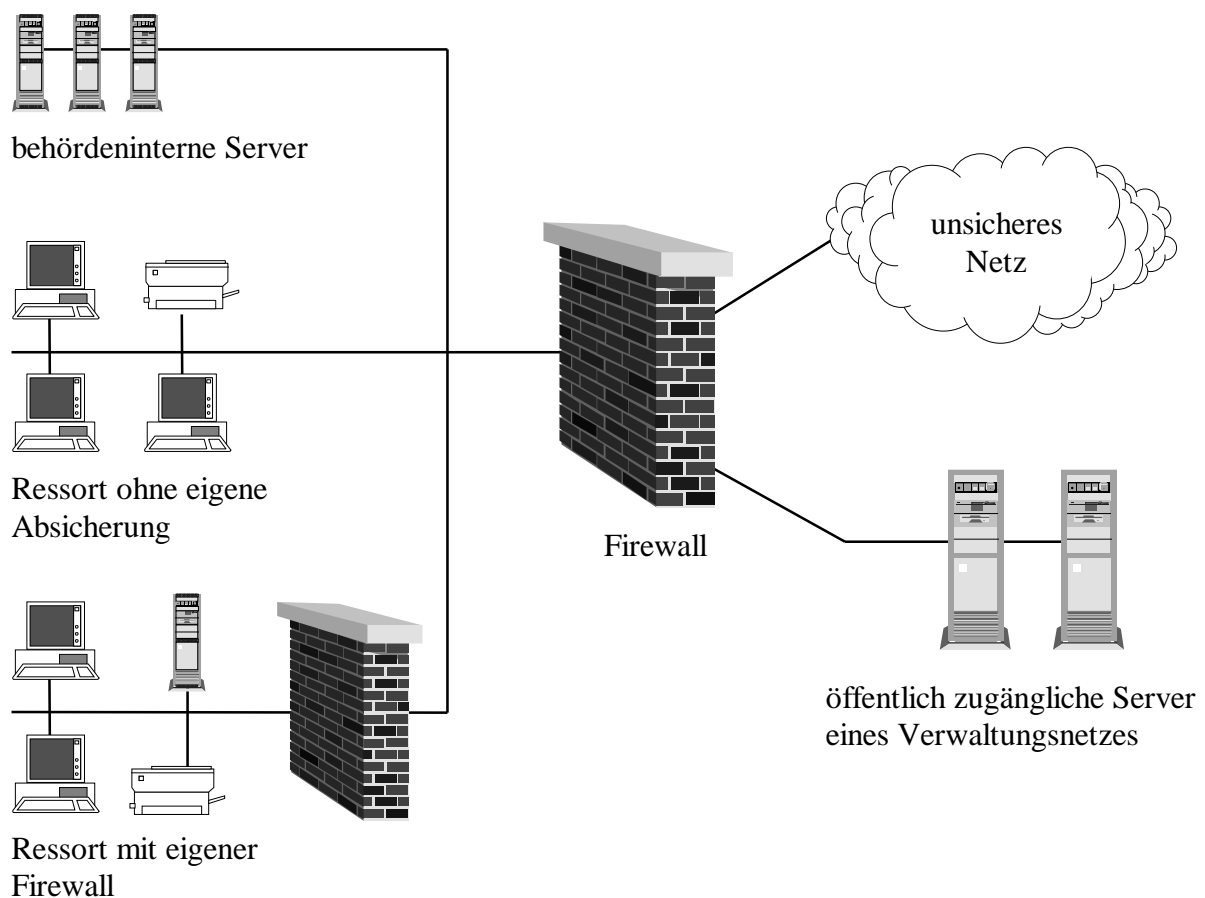
Abbildung 3.2: Gestaffelte Firewall-Anordnung
