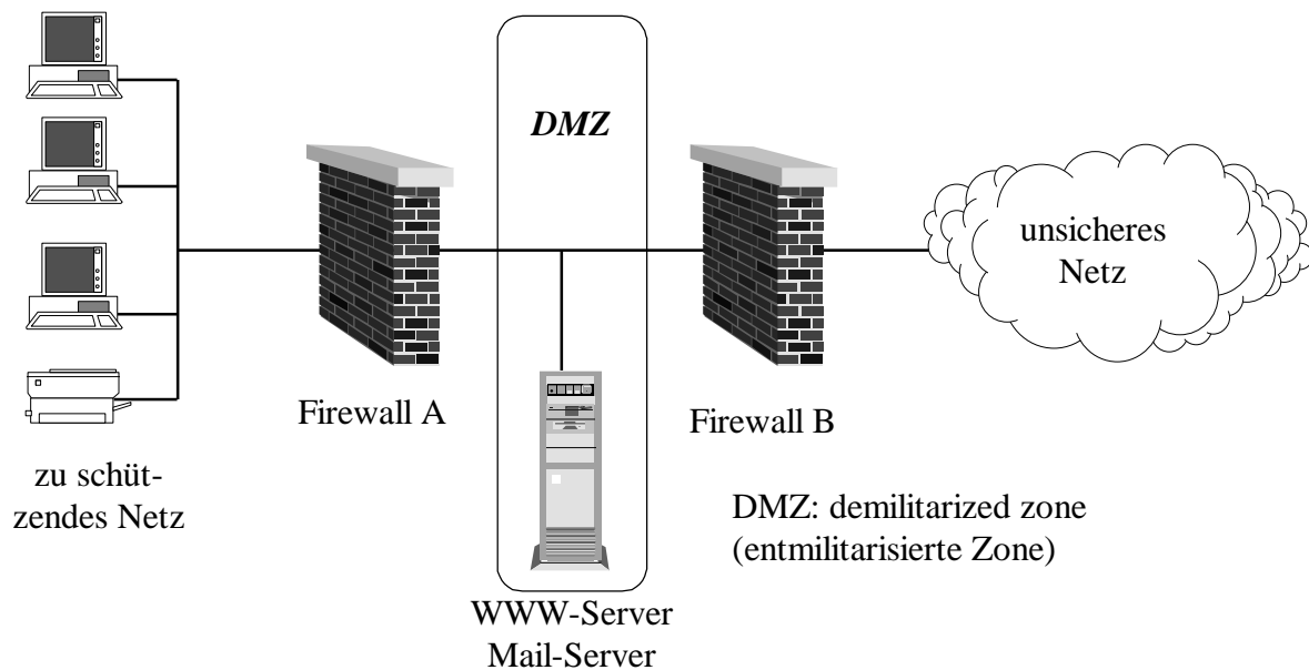
Abbildung 3.3: Kaskadierte Firewall-Anordnung mit DMZ
