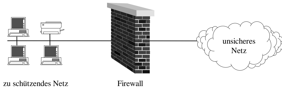
Abbildung 3.1: Zentrale Firewall-Anordnung
