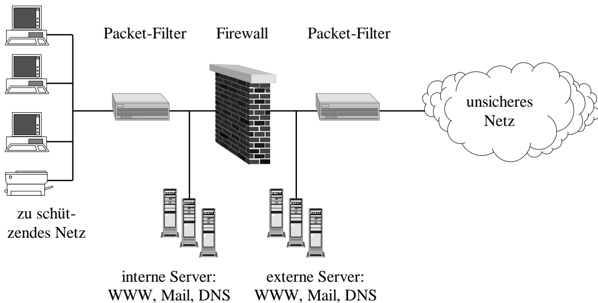
Abbildung 3.5: Screened Gateway (Sandwich-System) mit DMZ
